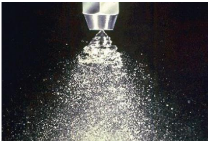
Κακή διάσπαση ψεκασμού
